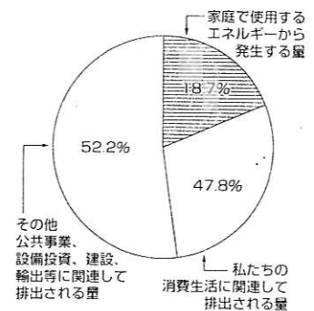
私たちの暮らしに関連して排出される二酸化炭素の占める割合
