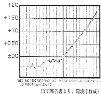
全世界の地表面気温の変化と予測
